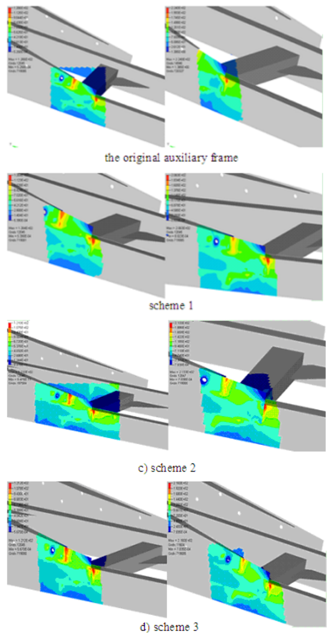
Fig. (9). A6 field stress nephogram.
