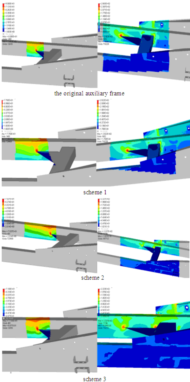
Fig. (8). A5 field stress nephogram.
